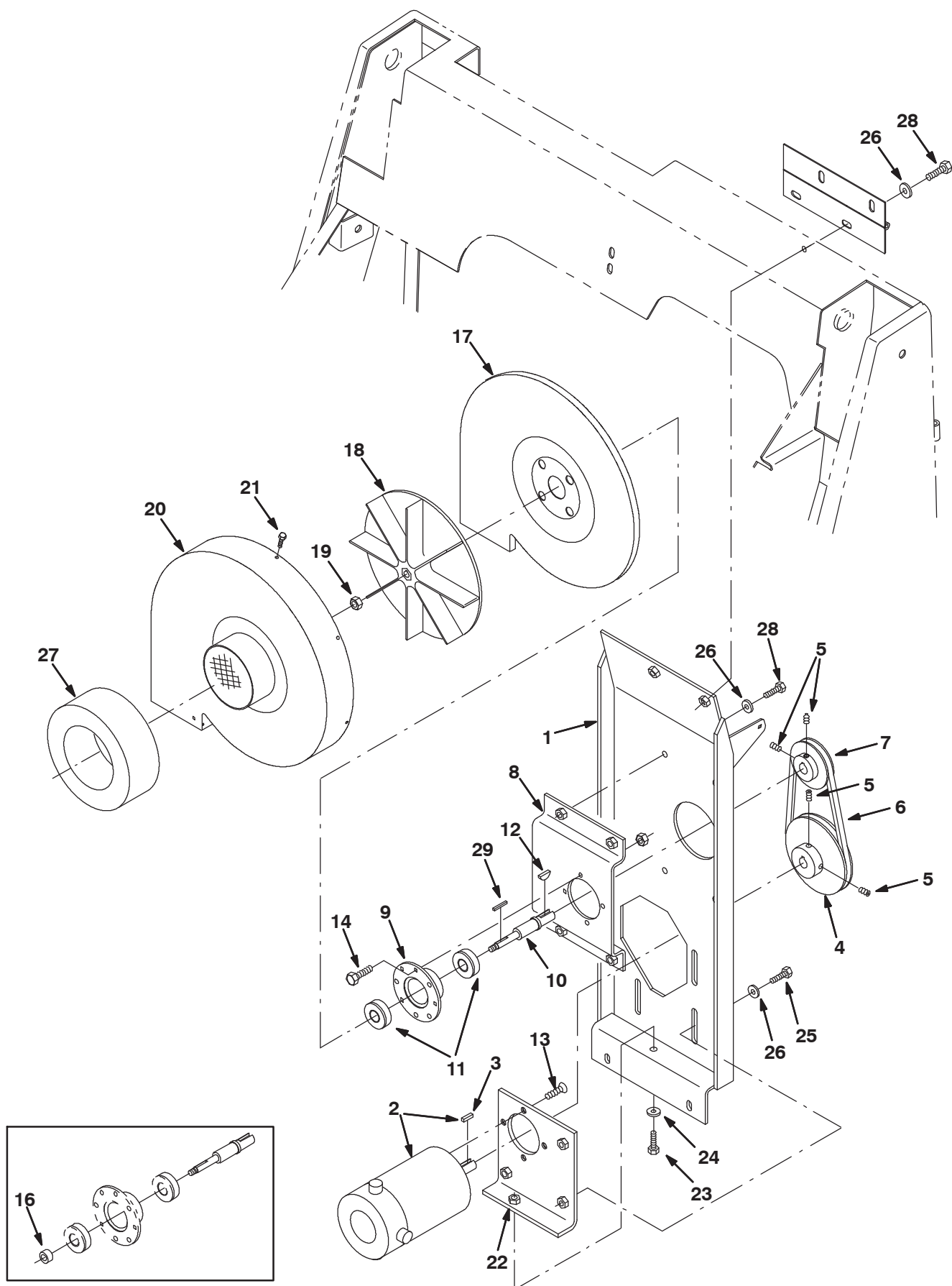
Fig. 50 - Sweeper Vacuum Fan Group
